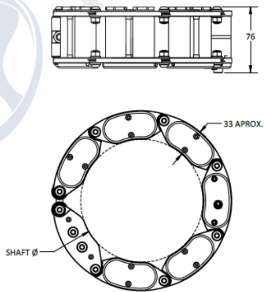
TTTS 转子尺寸(mm)
