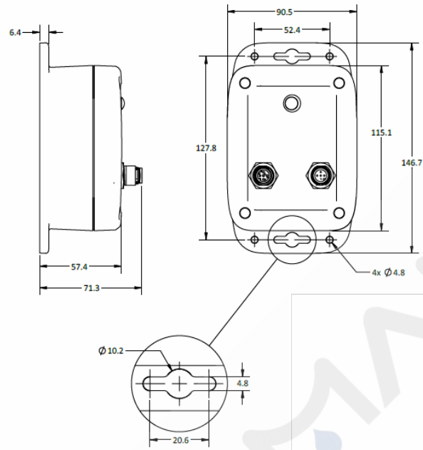
TTTS 接收机模块尺寸(mm)
